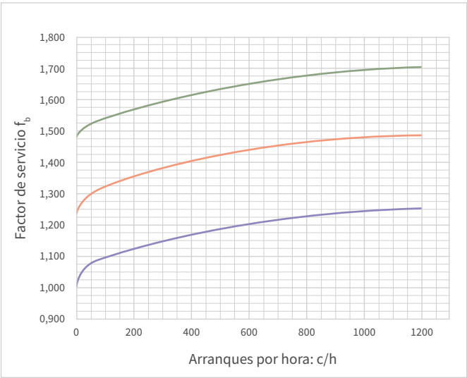
Determinación del factor de servicio f_b para 16 h/d de funcionamiento
