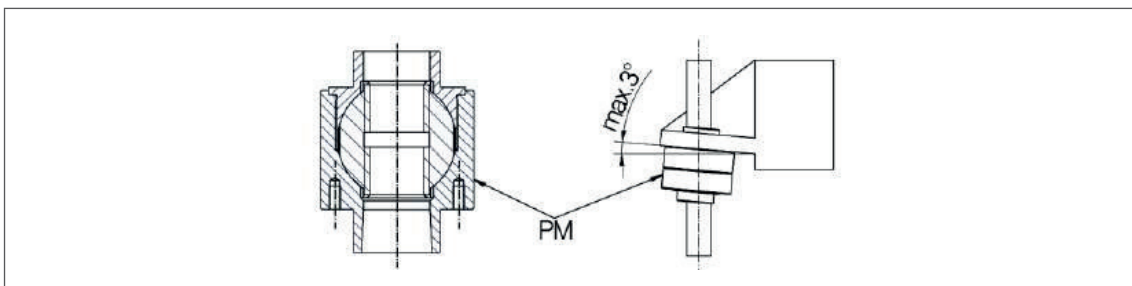
Fig. 10: Excepción: El ángulo máximo de inclinación de la tuerca oscilante (PM) es de 3°, monte todas las demás tuercas en ángulo recto.
